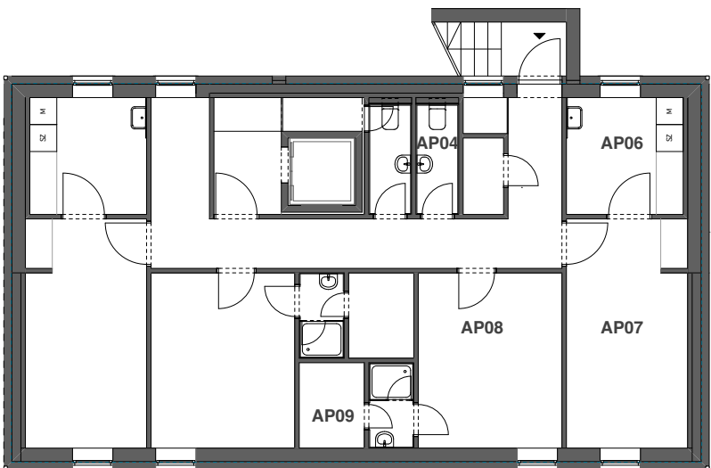
Pincszinti alaprajz
